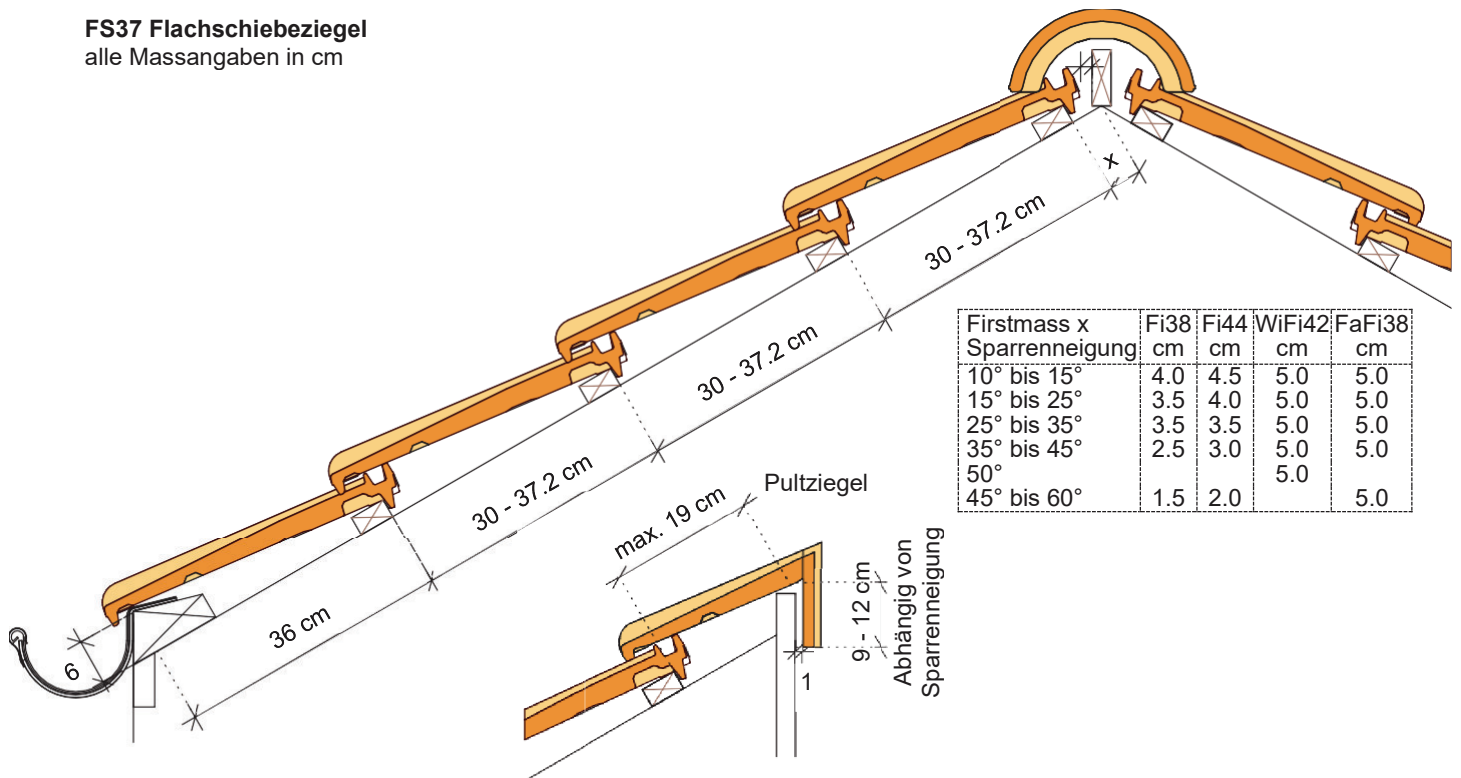
Flächenziegel
